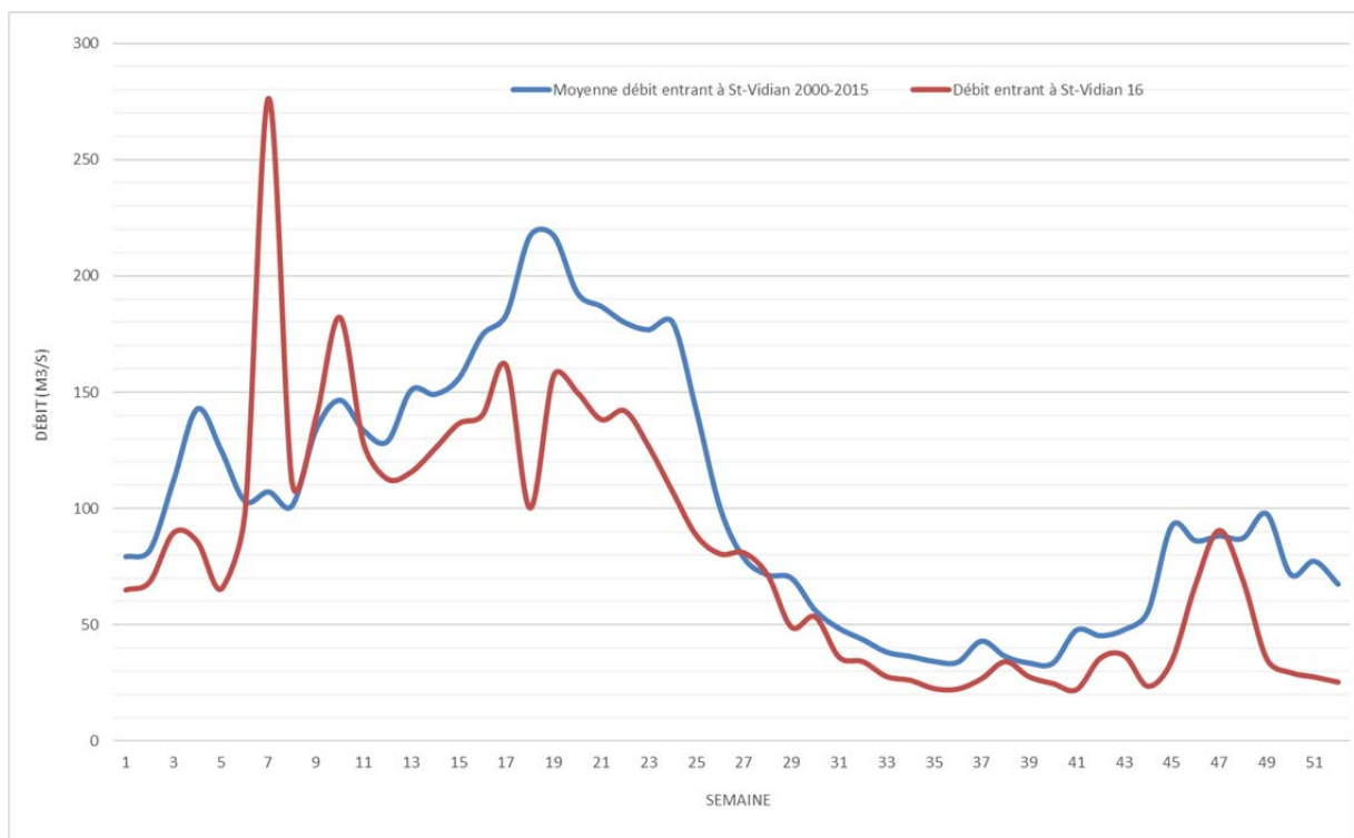
Figure 7 : Evolution du débit de la Garonne en amont de Carbonne (St Vidian) entre le 1/01/16 et le 31/12/16. Comparaison avec la moyenne de 2000 à 2015
