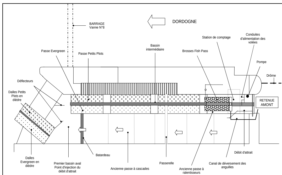
Figure 10 : Schéma du dispositif de franchissement spécifique anguilles de Tuilières de 1997 à 2005
