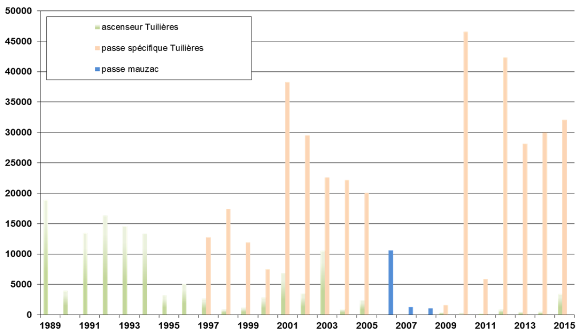
Figure 16 : Nombre d'anguilles passées à Tuilières en 2015
