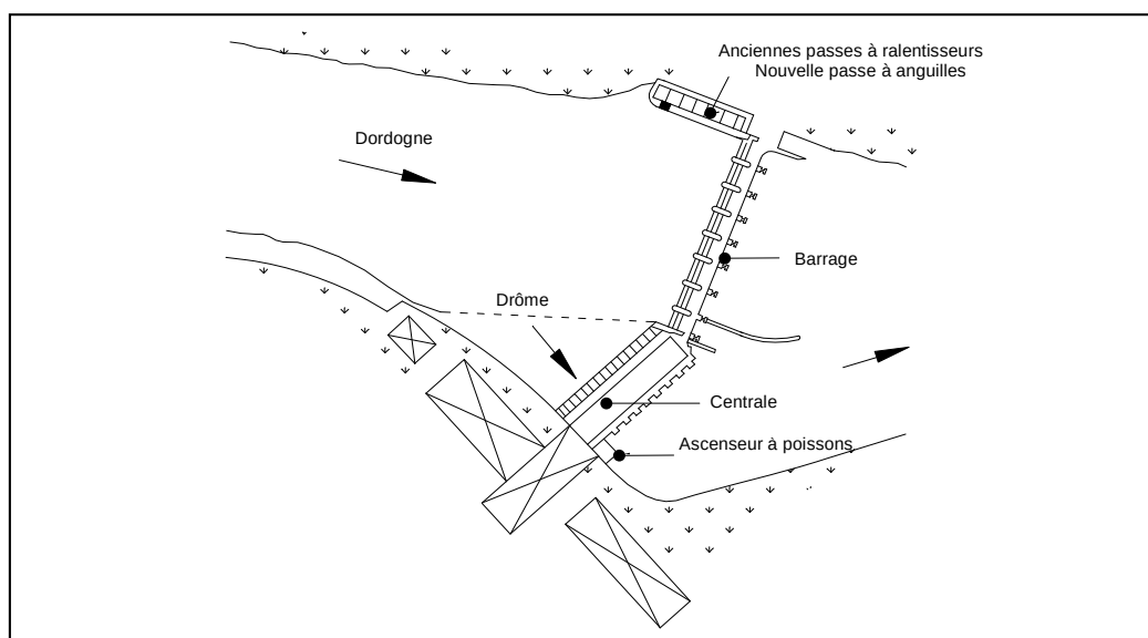
Figure 9 : Localisation de la passe à anguilles sur le site de Tuilières
