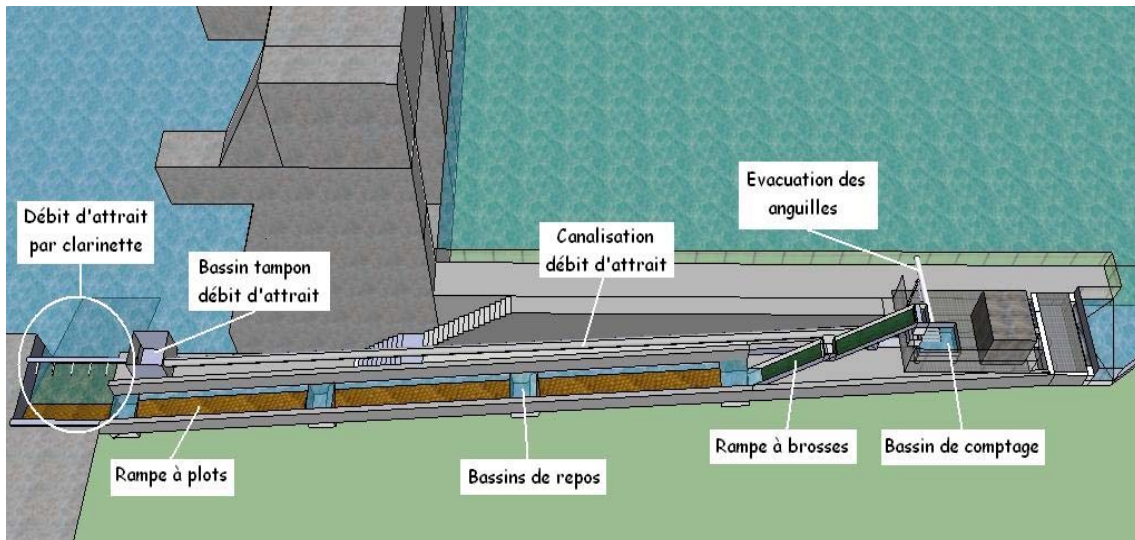
Figure 15 : Schéma de situation de la passe installée depuis 2010 sur le site de Tuilières
