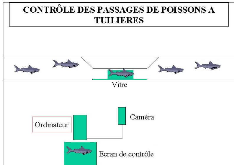
Photo 6 : Principe du système de vidéo surveillance de Tuilières
