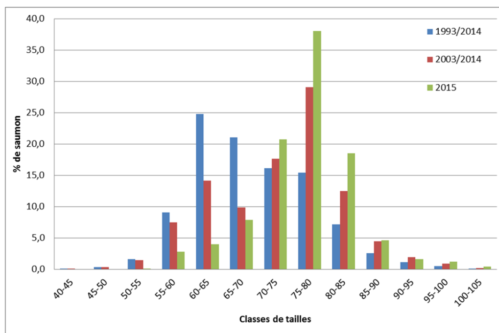
Figure 26 : Comparaison des histogrammes des classes de tailles moyennes de saumons à Tuilières/Mauzac entre 1993 et 2014, et celles observées à Tuilières en 2015
