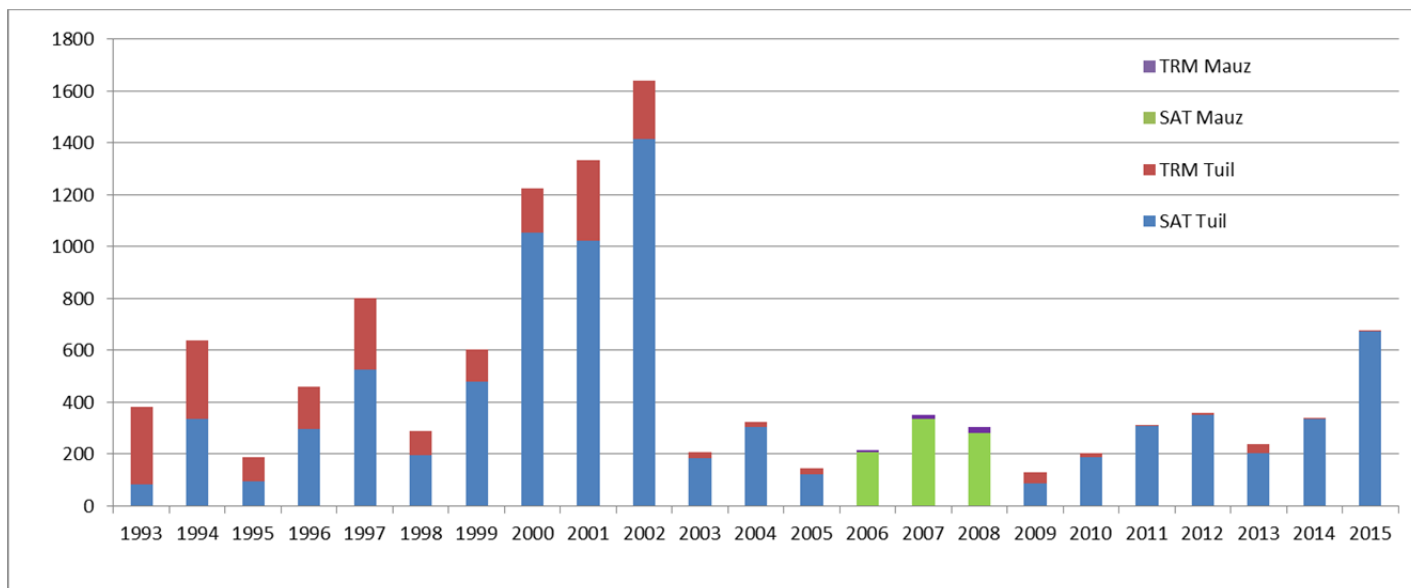
Figure 23 : Passages annuels des grands salmonidés à Tuilières et Mauzac entre 1993 et 2015
