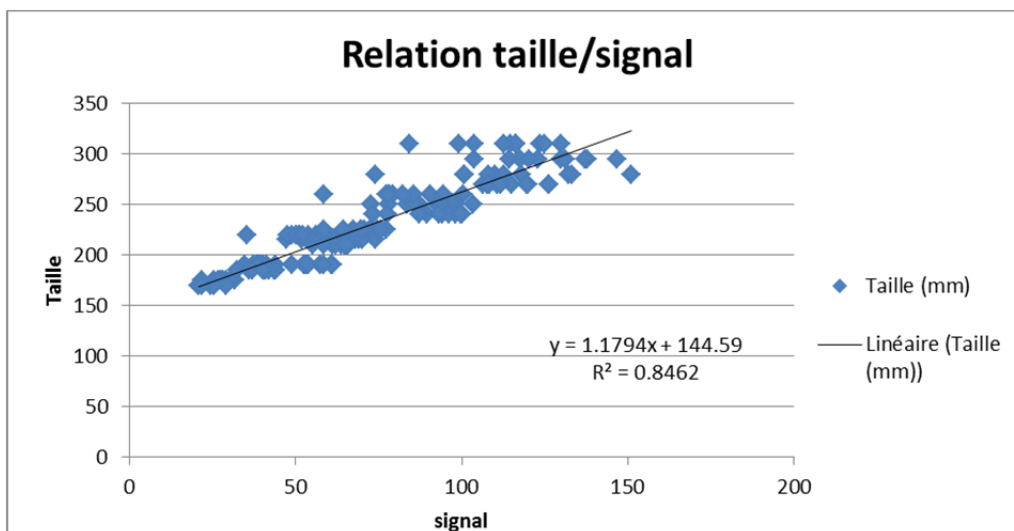
Figure 21 : Relation entre la taille des individus et le signal du compteur à Tuilières en 2015
