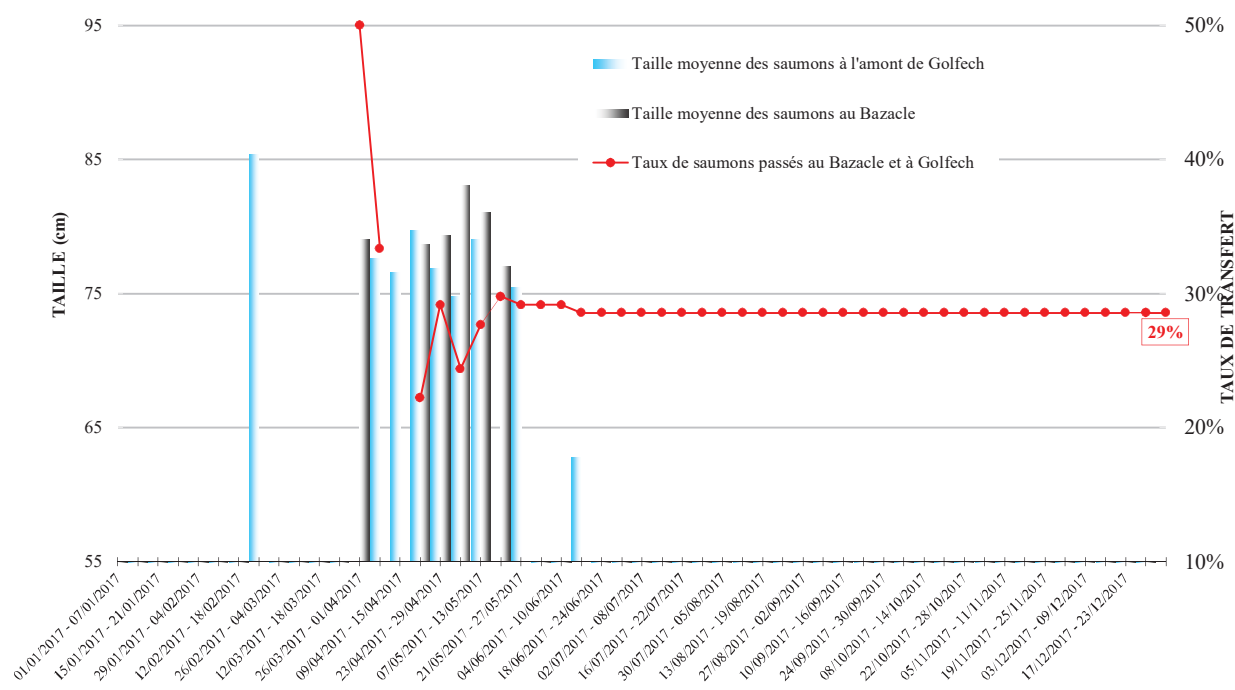
FIGURE 14 : EVOLUTION PAR SEMAINE DU TAUX DE TRANSFERT DES SAUMONS ENTRE GOLFECH ET LE BAZACLE, ET DE LA TAILLE MOYENNE EN 2017
