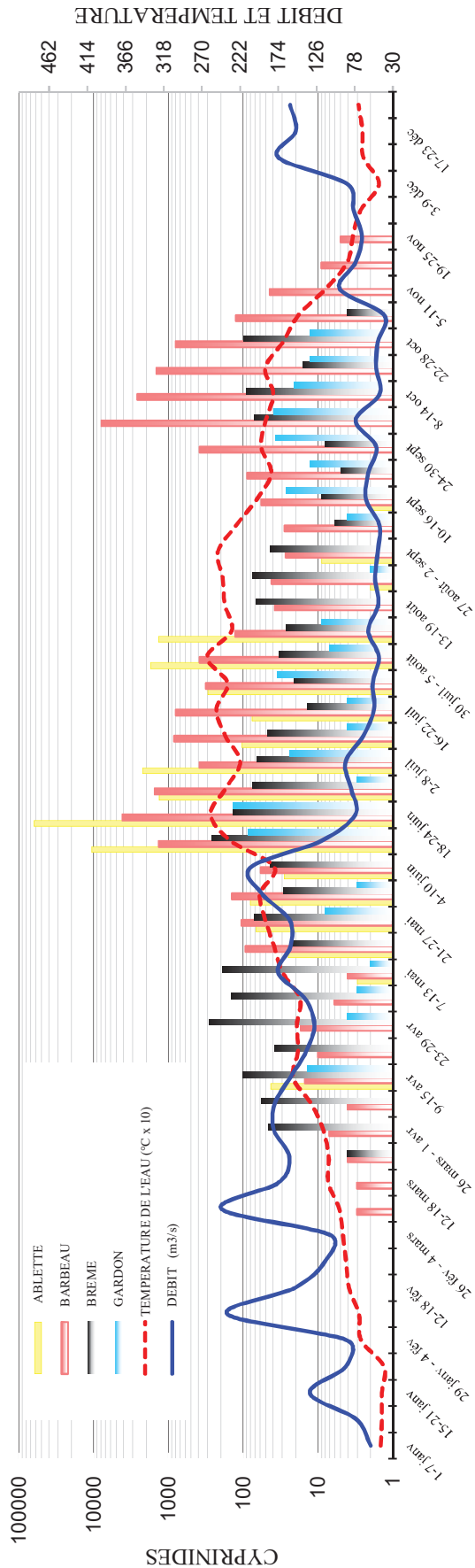
FIGURE 11 : MIGRATIONS DES CYPRINIDES ET CONDITIONS ENVIRONNEMENTALES AU BAZACLE EN 2017
