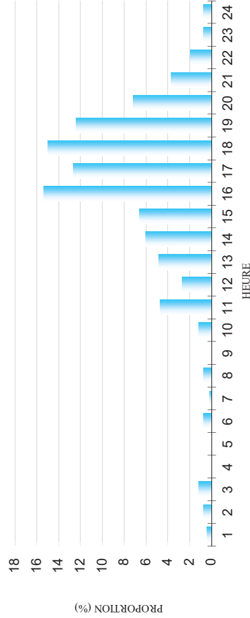
ACTIVITE HORAIRE DES GARDONS AU BAZACLE EN 2017
