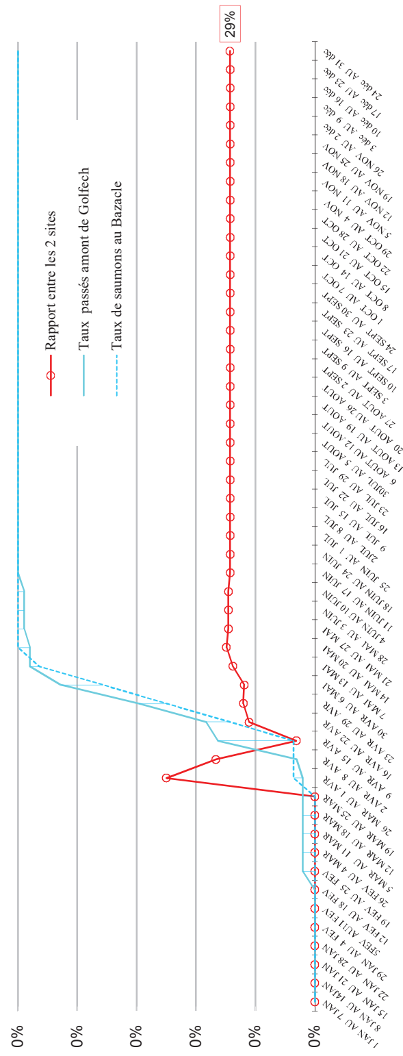
FIGURE 13 : FONCTIONNEMENT DE GOLFECHET COMPARAISON DES PASSAGES CUMULES DES SAUMONS PASSES A L'AMONT DE GOLFECHET AU BAZACLE EN 2017
