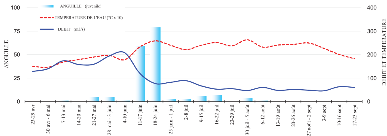
FIGURE 8 : HISTOGRAMME DES TAILLES DES ANGUILES AU BAZACLE EN 2017
