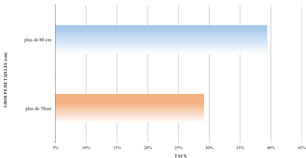
FIGURE 15 : TAUX DE TRANSFERT DES SAUMONS ENTRE GOLFECH ET LE BAZACLE SELON LE GROUPE DE TAILLES EN 2017
