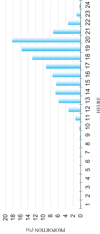
ACTIVITE HORAIRE DES ABLETTES AU BAZACLE EN 2017
