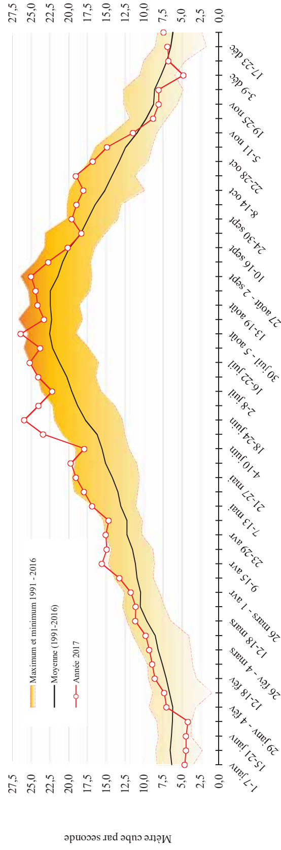
FIGURE 5 : COMPARAISON DES TEMPERATURES DE L'EAU EN GARONNE AU BAZACLE DEPUIS 1991
