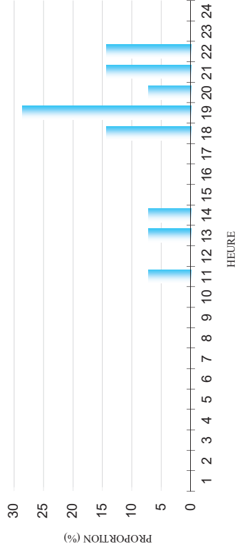
ACTIVITE HORAIRE DES SAUMONS AU BAZACLE EN 2017
