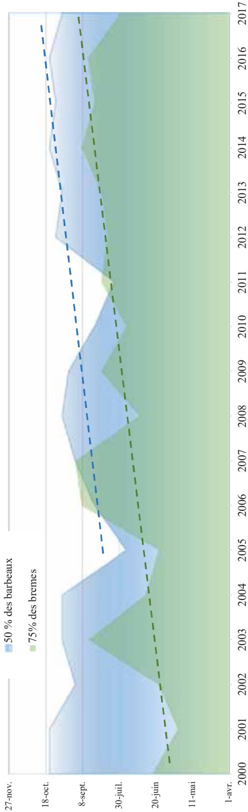
Figure 11.1 : Evolution de la date des passages des migrations de barbeaux et de bremes au Bazacle
