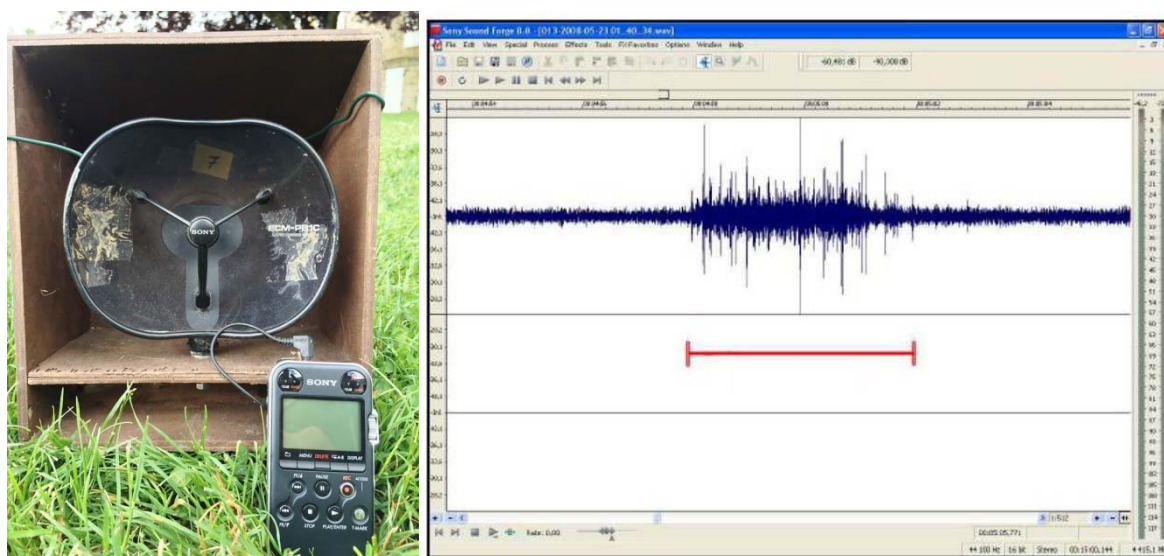
Figure 4 : Dispositif d'enregistrement et spectre audio d'un bull
