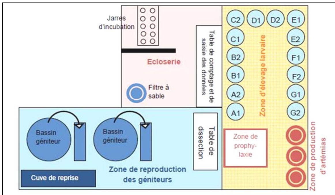
Figure 6 : Organisation des structures dans le local de production.
