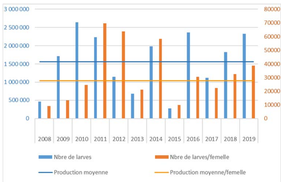
Figure 22: Synthèse des productions totales par année depuis 2008 et des productions par femelle
