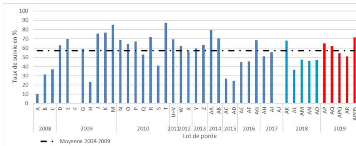
Figure 18 : Taux de survie à l'incubation des pontes par lot de géniteurs et par année
