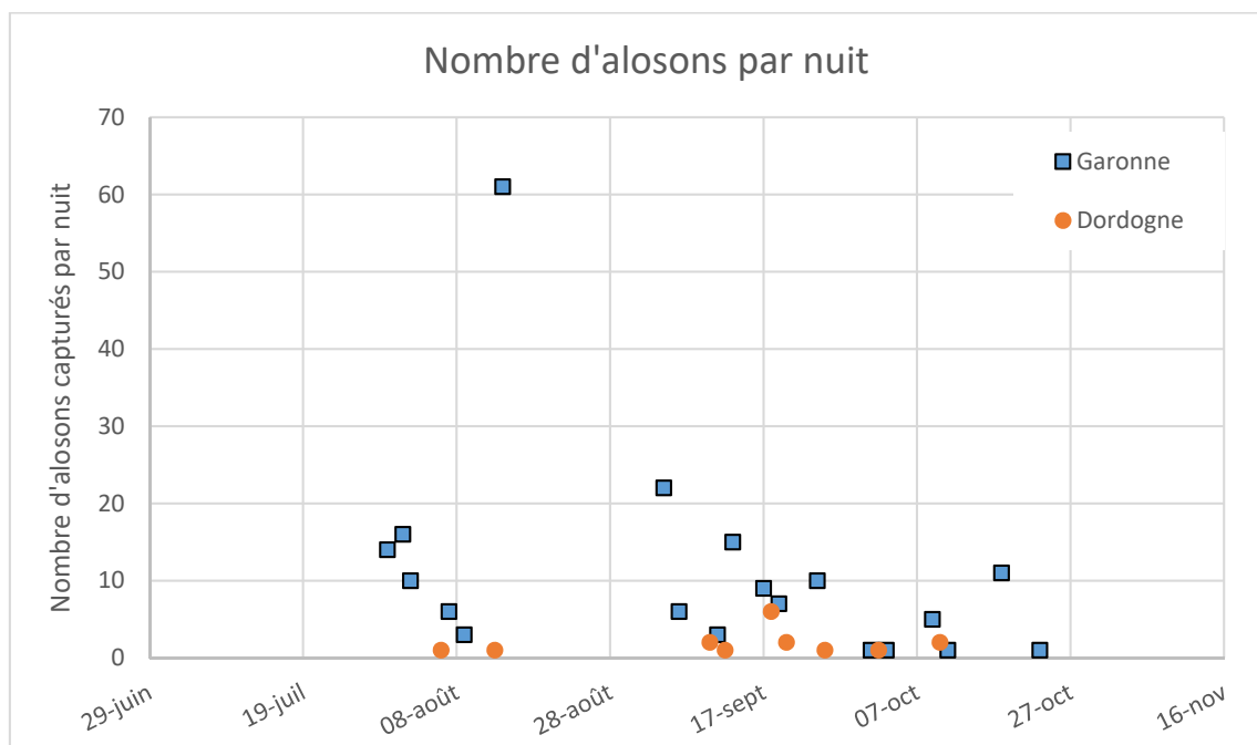
Figure 36 : Captures de juvéniles de grande alose au cours de la saison sur les deux rivières en 2019
