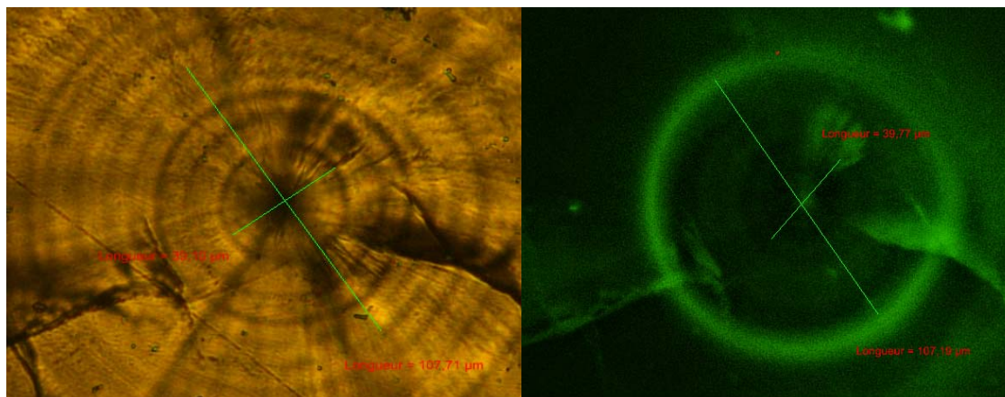
Figure 42 : Photographie d'un otolithe d'aloson marqué en coupe sagittale sous lumière blanche et sous éclairage fluorescent (440 nm)
