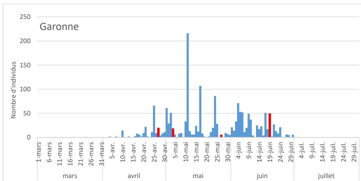
Figure 12 : Effectifs journaliers d'individus ayant franchi le barrage de Golfech en 2019. Piégeage en rouge.
