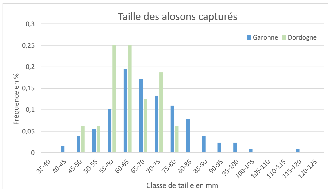
Figure 38 : Histogramme des tailles des alosons capturés à Marmande et Pessac sur Dordogne
