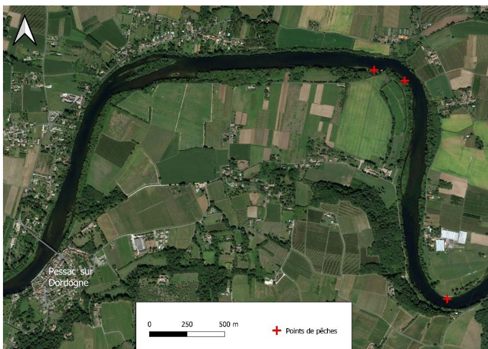
Figure 33 : Sites de pêches au niveau de Pessac sur Dordogne
