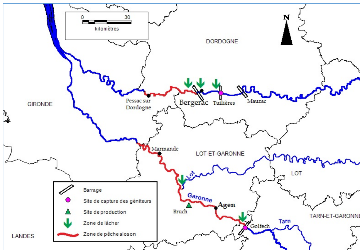
Figure 7 : Localisation géographique des activités de l'opération.
