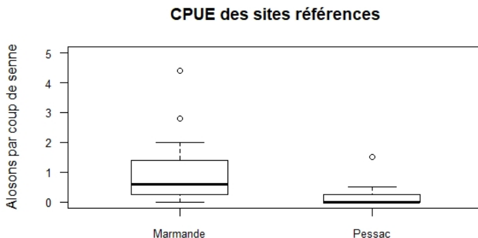
Figure 40 : Boxplot des CPUE des stations de référence en 2019
