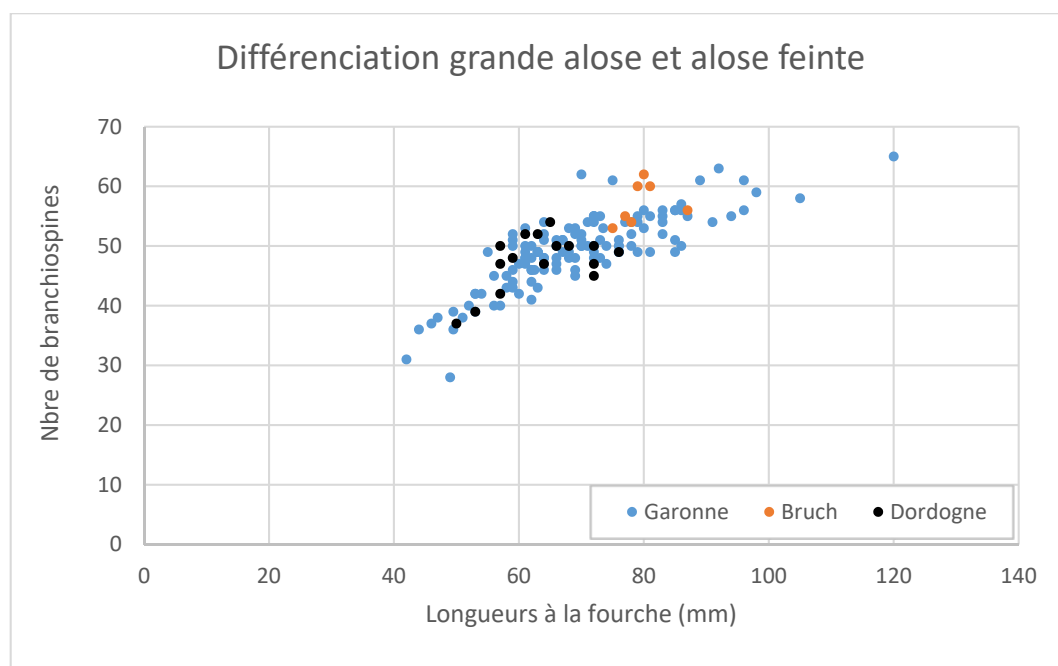
Figure 31 : Représentation du nombre de branchiospines des alosons en fonction de la taille
