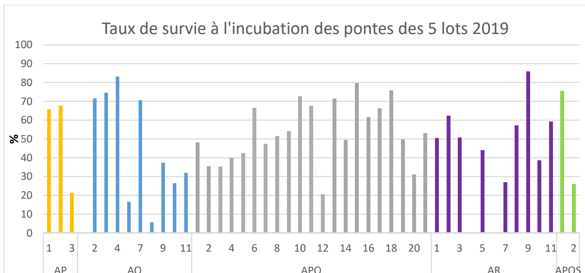
Figure 17 : Taux de survie à l'incubation de chacune des pontes des lots AP, AQ, APQ, AR et APQS récoltées en 2019.
