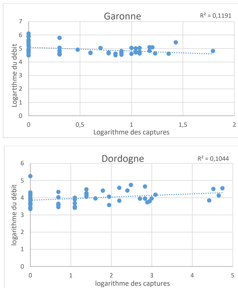
Figure 37 : Relation (\ln + 1) entre les débit et les captures des alosons sur la Garonne et la Dordogne. Données 2017, 2018 et 2019.
