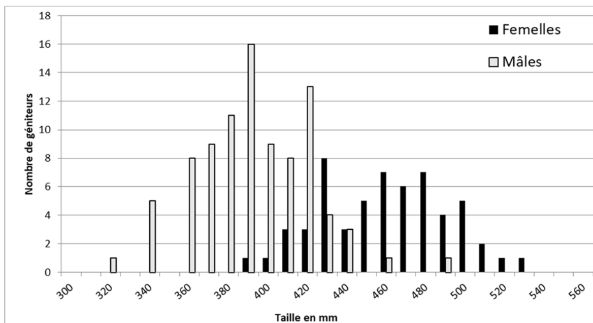
Figure 14 : Histogramme des tailles (longueur fourche en mm) des géniteurs capturés en 2019 par sexe.
