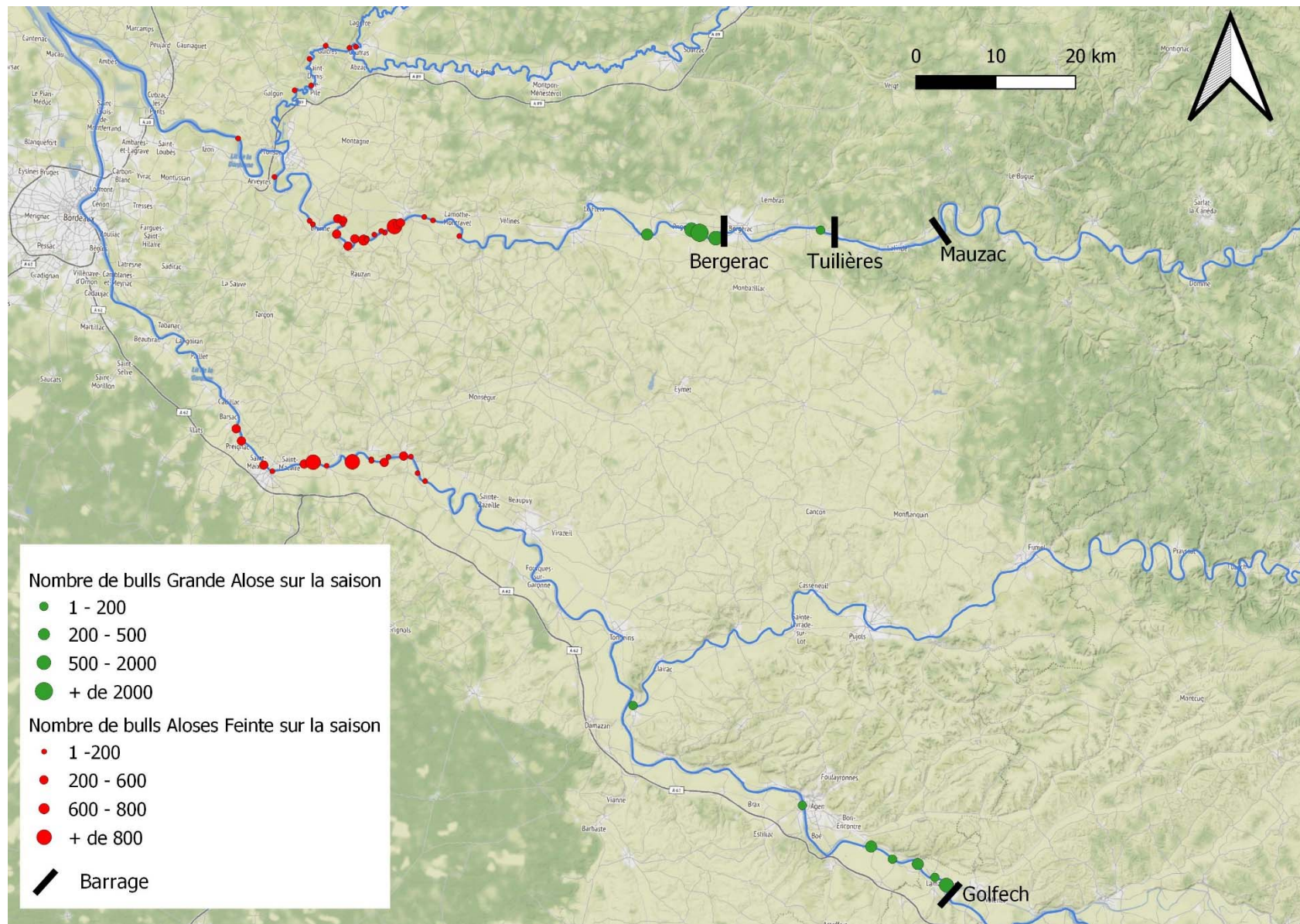
Figure 28 : Représentation cartographique de l'activité de reproduction sur frayère des aloses en Garonne-Dordogne en 2019.
