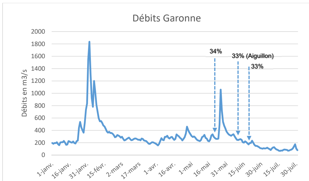
Figure 25 : Evolution du débit de la Garonne (en m³/s) à Golfech et pourcentage de larves lâchées selon la date.
