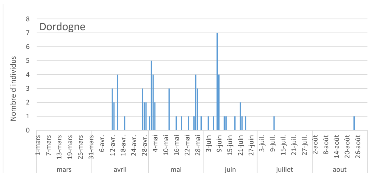
Figure 13 : Effectifs journaliers d'individus ayant franchi le barrage de Tuilières en 2019. Pas de piégeage.
