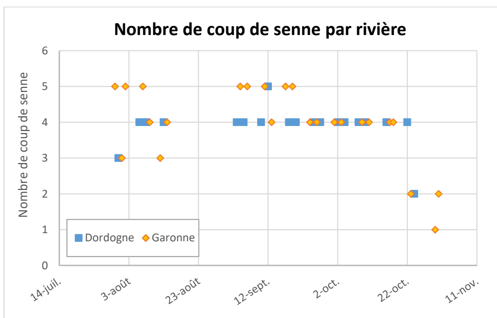
Figure 30 : Représentation du nombre de coups de senne par nuit d'échantillonnage sur la Garonne et la Dordogne.
