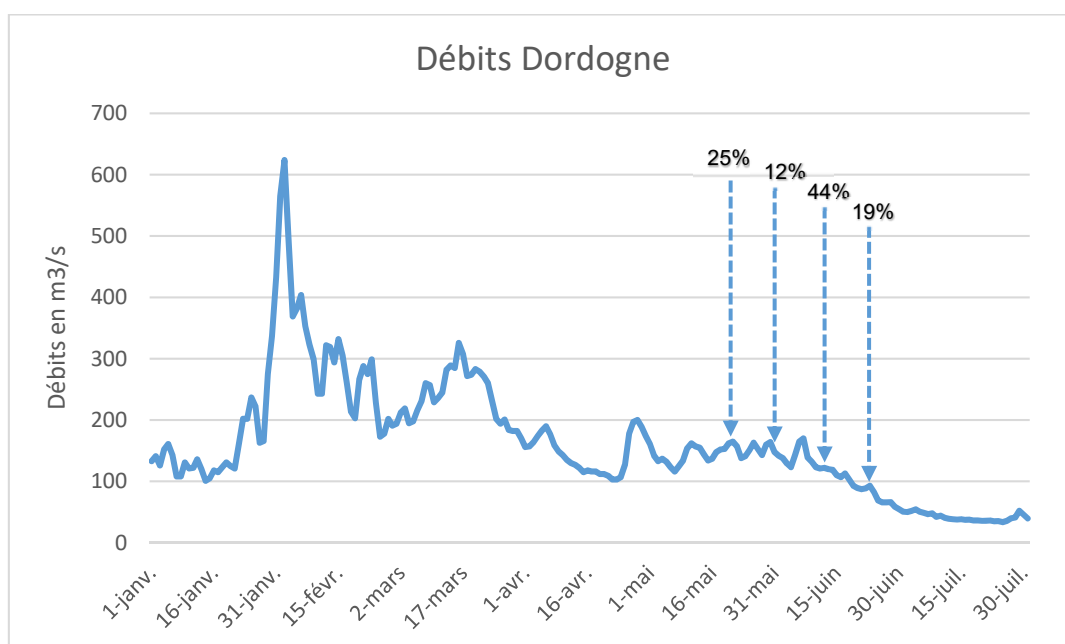
Figure 26 : Evolution du débit de la Dordogne à Lamonzie St Martin (en m³/s) et pourcentage de larves
