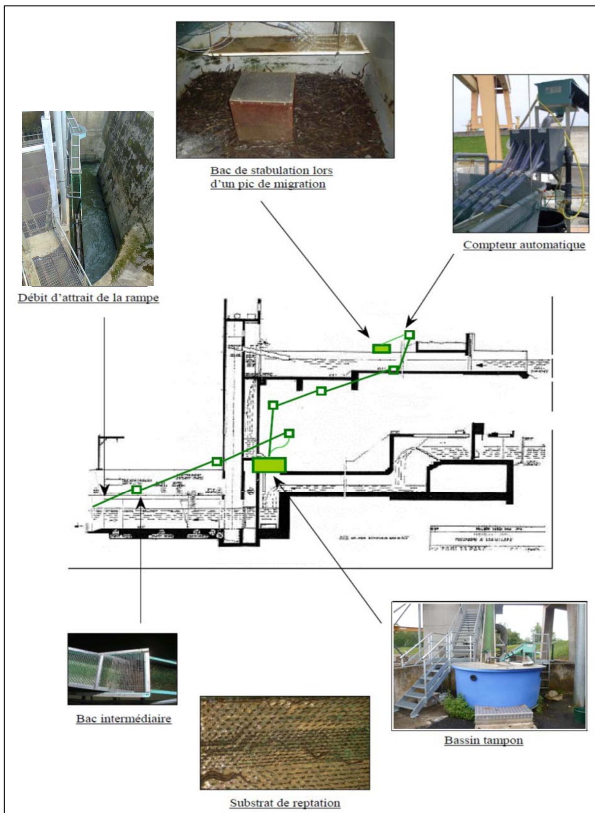
Figure 52 : Schéma de la rampe à anguilles définitive
