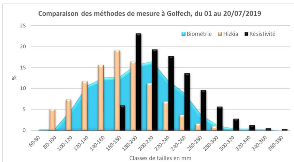
Figure 60 : Comparaison de la répartition des classes de tailles selon les 3 méthodes de mesures : manuelles, compteur à résistivité, Système hizkia
