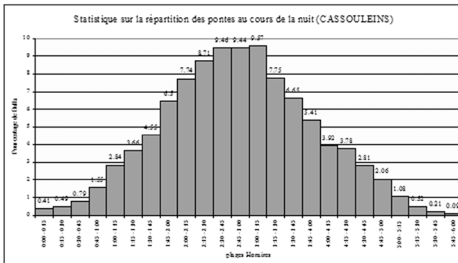
Figure 38 : Modèle statistique sur la répartition des pontes au cours de la nuit (CASSOU-LEINS, 1985)
