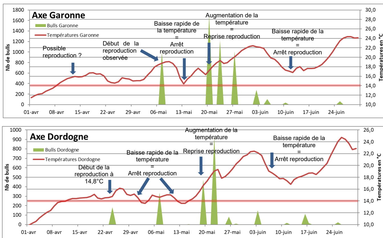
Figure 17 : Evolution de l'activité de reproduction par rapport à la température de l'eau en 2020 (en rouge seuil des 14°C)
