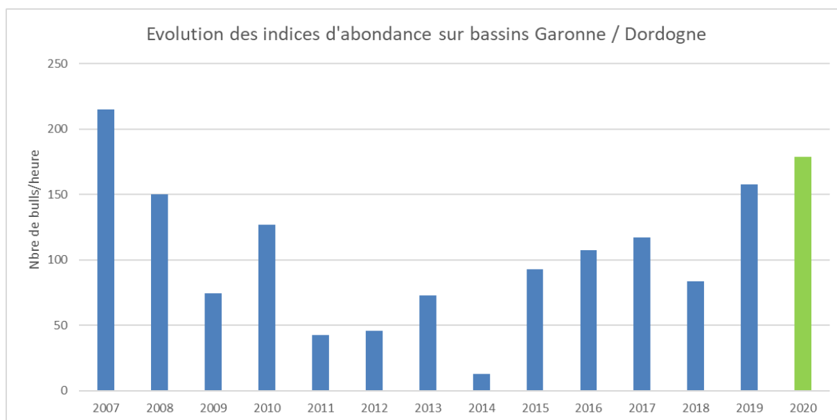
Figure 21 : Indicateur d'abondance de la population d'alose feinte
