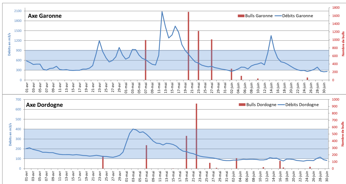
Figure 16 : Evolution de l'activité de reproduction par rapport aux débits sur les bassins Garonne Dordogne en 2020 (bande bleu : préférendum de débits pour l'espèce)
