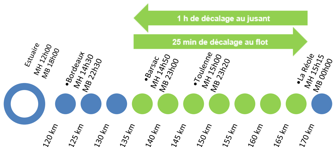
Figure 19 : Représentation du décalage de la marée entre la pointe de Grave et La Réole (les zones favorables à la reproduction sont en vert)
