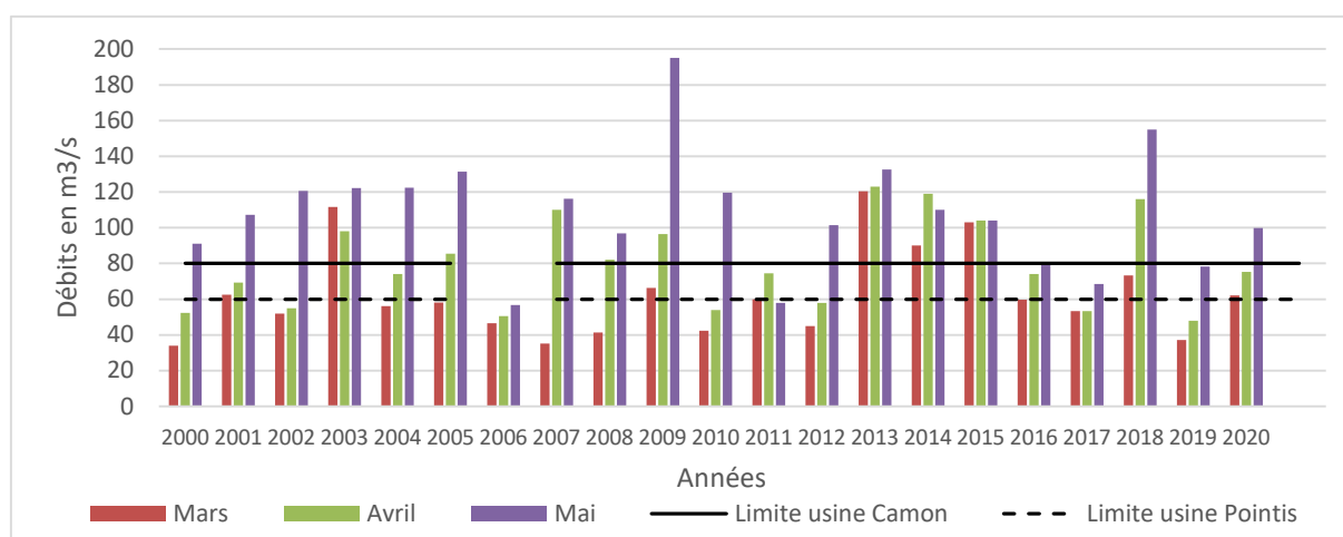
Figure 12 : Comparaison des débits journaliers de la Garonne mesurés à Valentine ou à Gourdan-Polignan de 2000 à 2020 (en pointillé niveau d'équipement des centrales)
