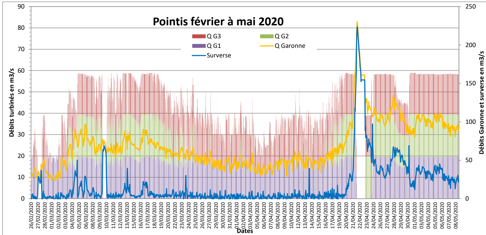
Figure 5 : Fonctionnement des groupes de l'usine de Pointis et débit de la Garonne durant la campagne 2020 (débit en m 3 /s)
