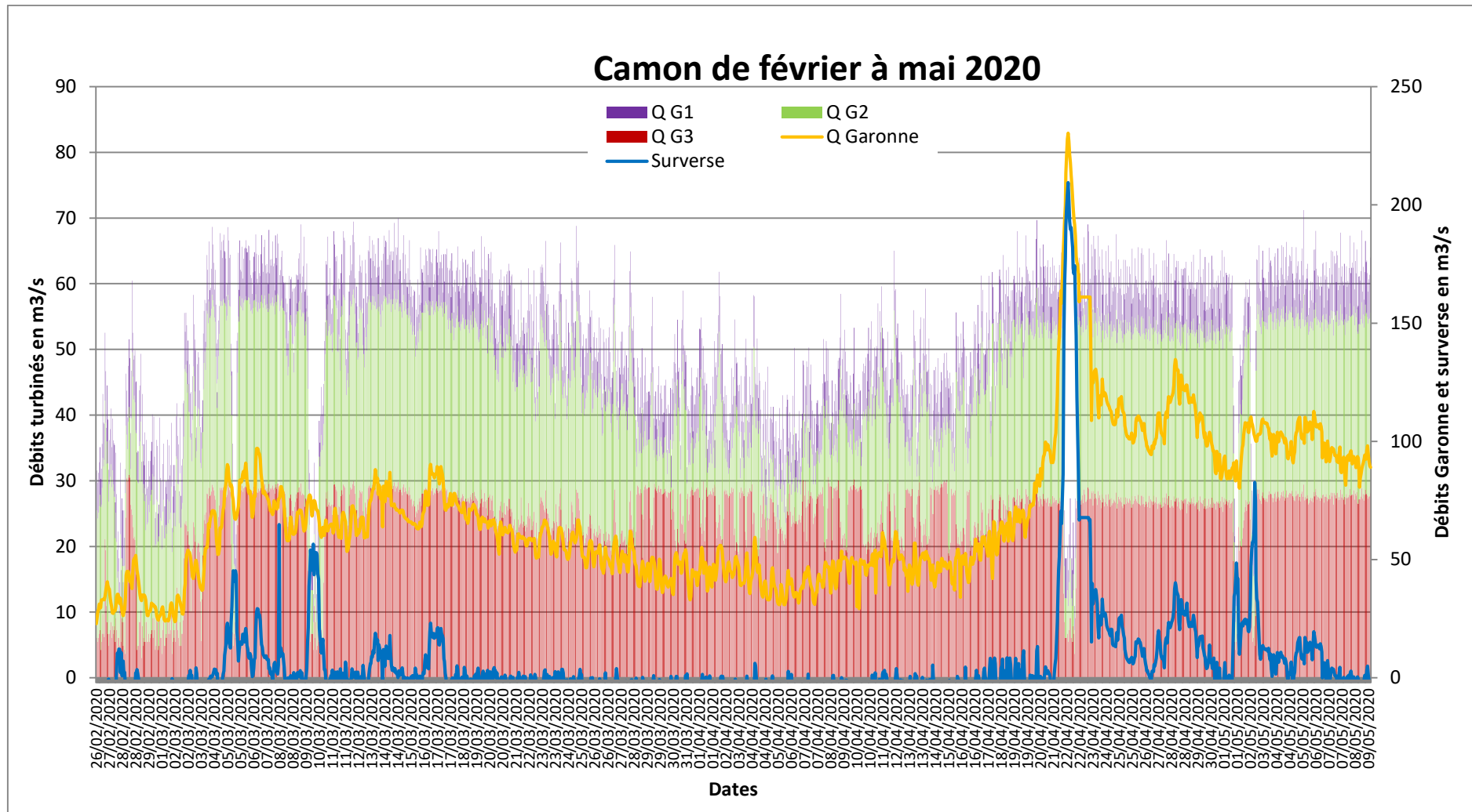
Figure 4 : Fonctionnement des groupes de l'usine de Camon et débit de la Garonne durant la campagne 2020 (débit en m³/s)
