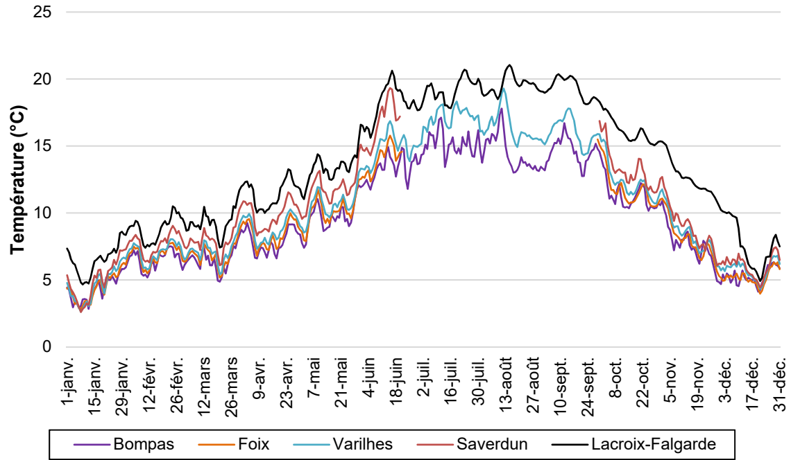
Figure 2 : Evolution des températures moyennes journalières sur l'Ariège en 2022
