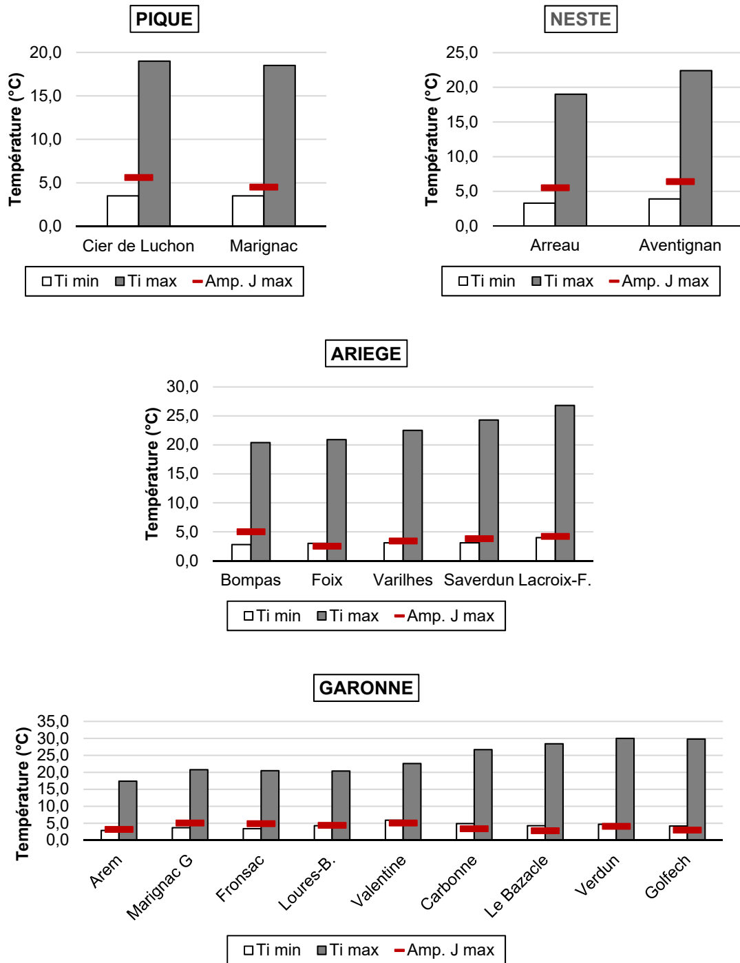
Figure 6 : Températures instantanées minimales, maximales et amplitudes journalières maximales enregistrées sur les stations suivies en 2022
