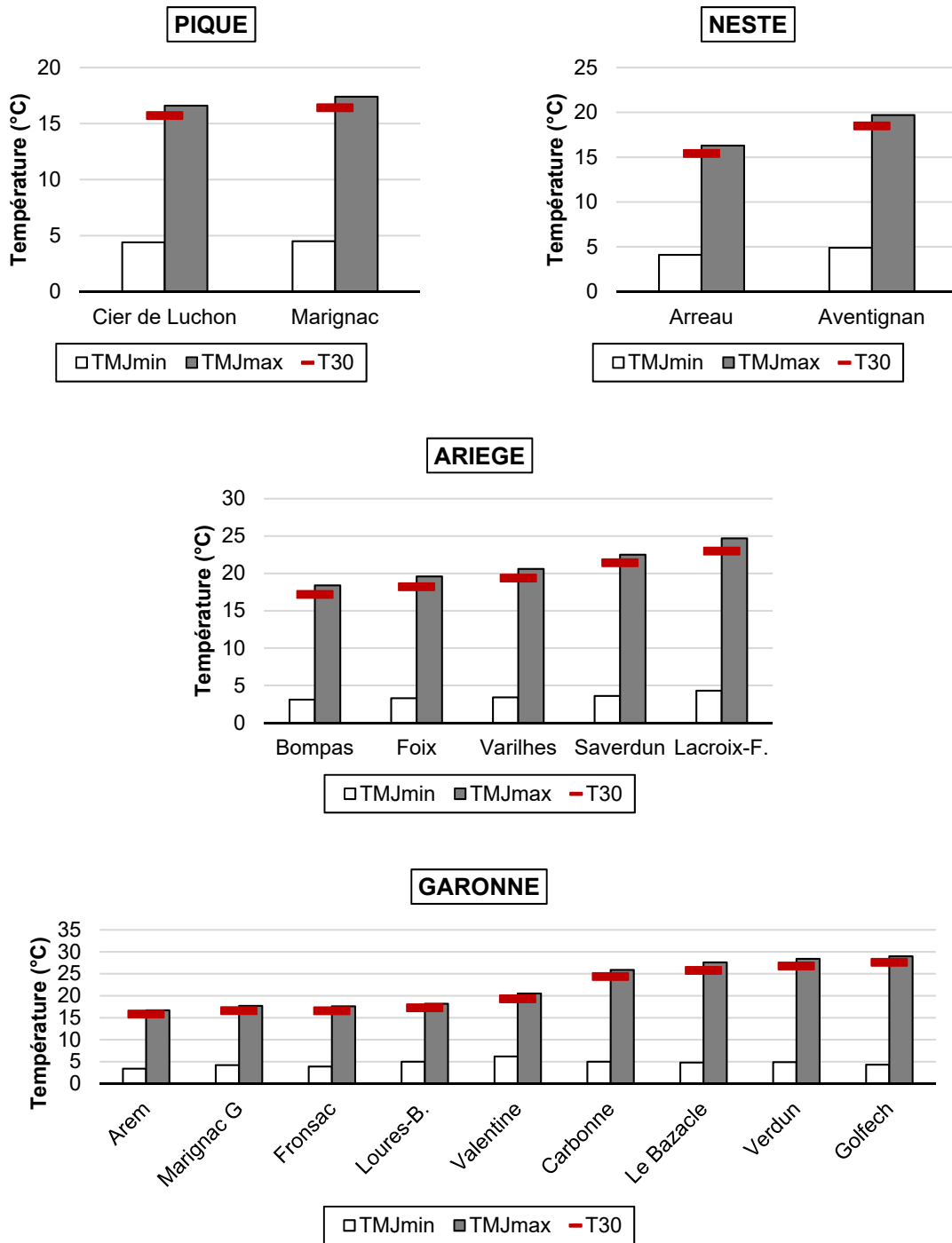
Figure 7 : Températures journalières moyennes minimales, maximales et moyenne des 30 jours consécutifs les plus chauds sur les stations suivies en 2022
