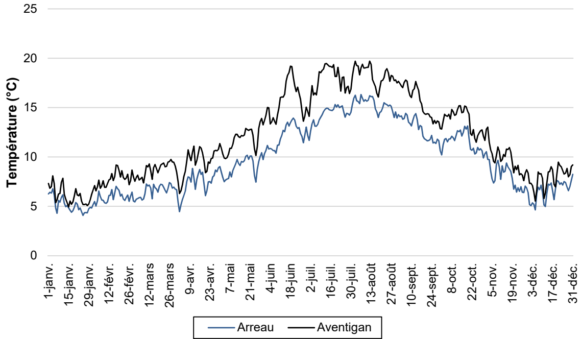
Figure 4 : Evolution des températures moyennes journalières sur la Neste en 2022
