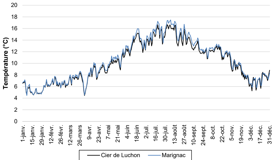
Figure 5 : Evolution des températures moyennes journalières sur la Pique en 2022
