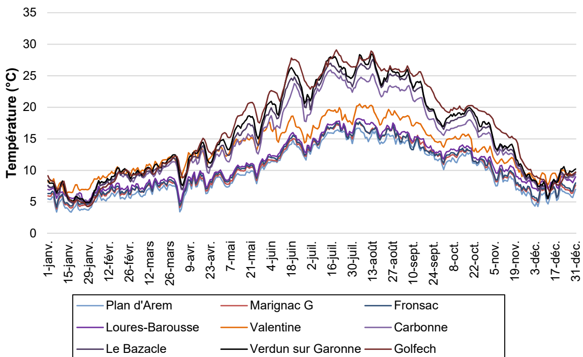
Figure 3 : Evolution des températures moyennes journalières sur la Garonne en 2022
