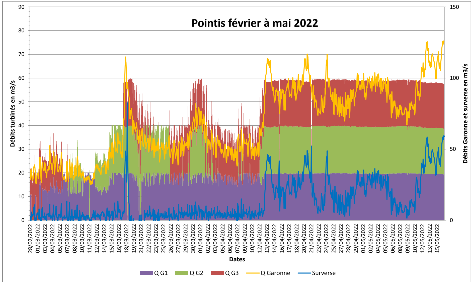
Figure 5 : Fonctionnement des groupes de l'usine de Pointis et débit de la Garonne durant la campagne 2022 (débit en m 3 /s)
