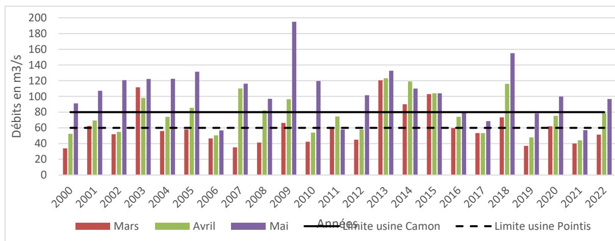
Figure 12 : Comparaison des débits journaliers de la Garonne mesurés à Valentine ou à Gourdan-Polignan de 2000 à 2022 (en pointillé niveau d'équipement des centrales)
