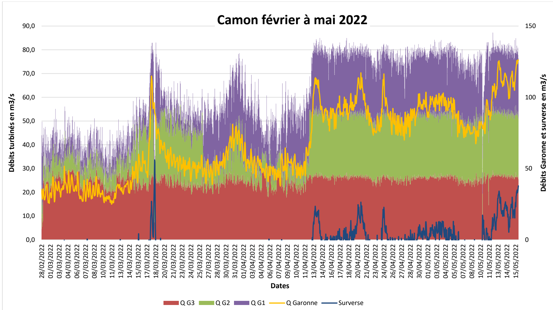
Figure 4 : Fonctionnement des groupes de l'usine de Camon et débit de la Garonne durant la campagne 2022 (débit en m 3 /s)
