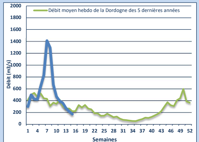
Débit moyen hebdomadaire de la Dordogne
