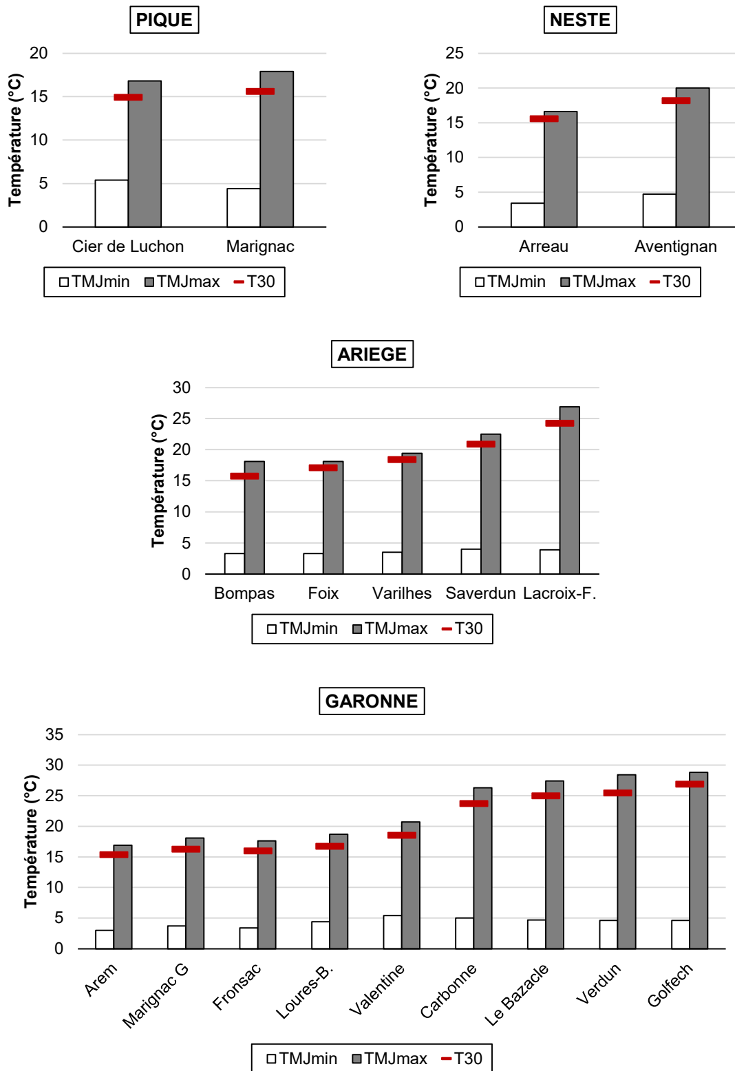
Figure 7 : Températures journalières moyennes minimales, maximales et moyenne des 30 jours consécutifs les plus chauds sur les stations suivies en 2025
