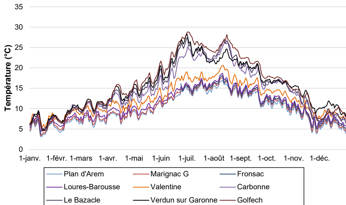
Figure 3 : Evolution des températures moyennes journalières sur la Garonne en 2025
