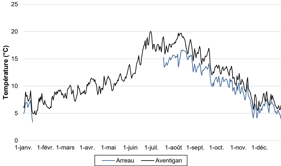
Figure 4 : Evolution des températures moyennes journalières sur la Neste en 2025
