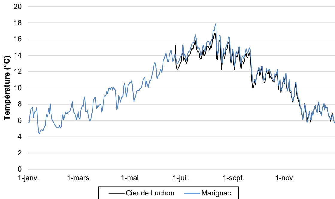
Figure 5 : Evolution des températures moyennes journalières sur la Pique en 2025
